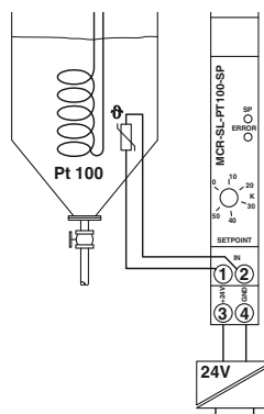
Пример использования - контроль температуры нагреваемой среды 1 - напряжение в сети
