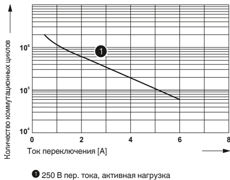
Срок службы электрических компонентов для PLC-RSP...UC/21RW
