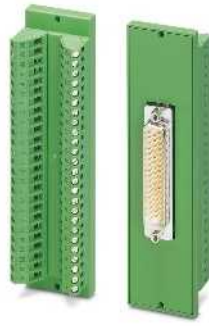
Со штыревой контактной частью разъема D-SUB
