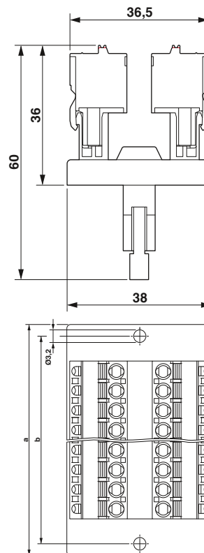
Чертеж DFLK...FKCT
