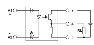
Рис. 4: 3-проводной выход
