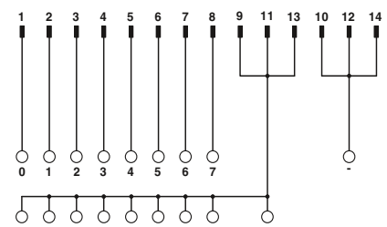
Схема подключения VIP-2/.../FLK14/8P/PLC
