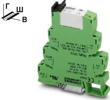
2 замыкающих контакта с силовым контактом
