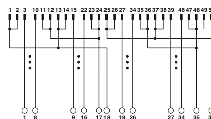
Схема подключения VIP-2/.../FLK50/AB-1756
