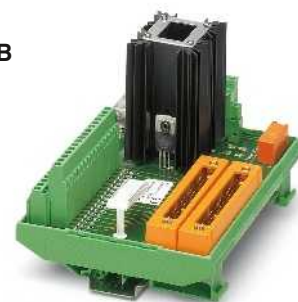
Пассивный интерфейсный модуль
