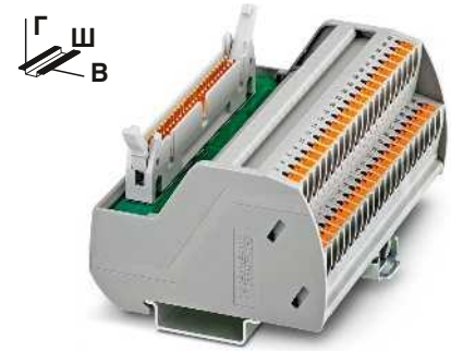
Пассивные интерфейсные модули для ввода-вывода, со специфической для SIMATIC® маркировкой и зажимом Push-in
