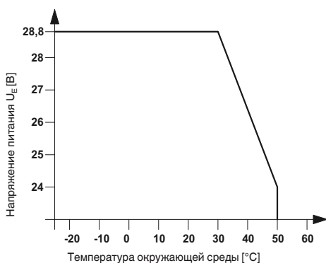
Кривая изменения характеристик для EIK 1-SVN 24 P
