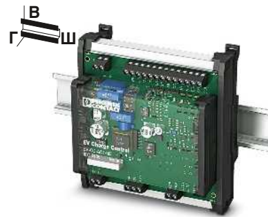
Управление зарядной в корпусе для установки на монтажную рейку
