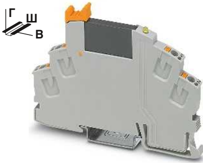
Выход постоянного напряжения, 100 мА
