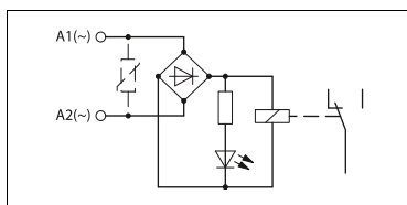
Принципиальная схема реле со входом переменного/постоянного тона
