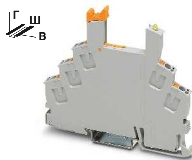
Релейный блок с 1 переключающим контактом для Миниатюрное силовое реле
