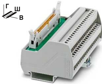
Пассивные интерфейсные модули для ввода-вывода, со специфической для SIMATIC® маркировкой и винтовым зажимом
