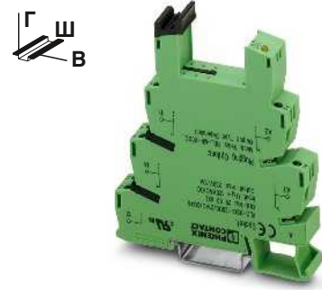
1 переключающий контакт для повышенных токов длительной нагрузки
