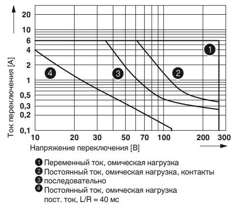
Мощность отключения для PLC-RSP...UC/21HC/RW
