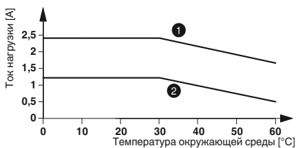
① = установлены в ряд с промежутком > 20 мм ② = установлены в ряд без промежутков
